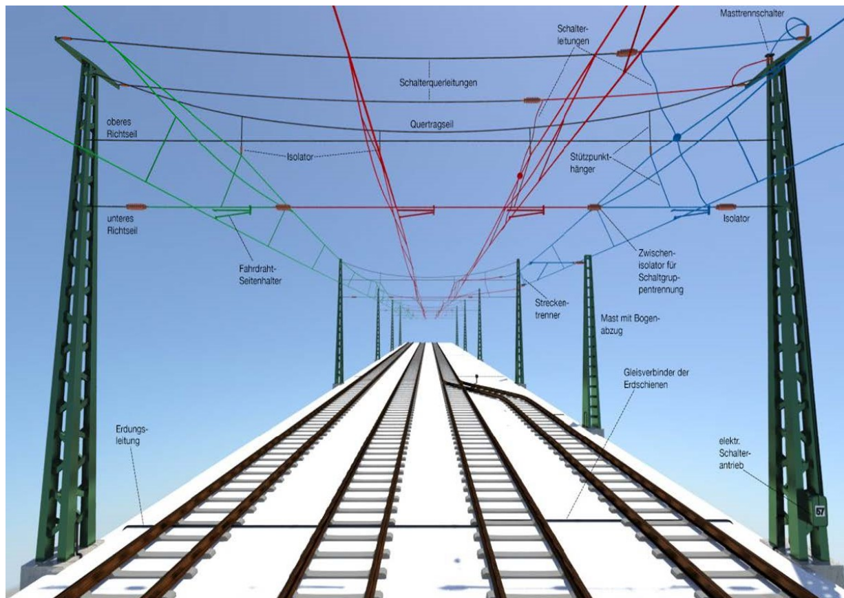
Abbildung 6: Oberleitung mit Querfeldern. Grün, blau und rot markieren unter Spannung stehende Anlagenteile (Quelle: DB Training)
