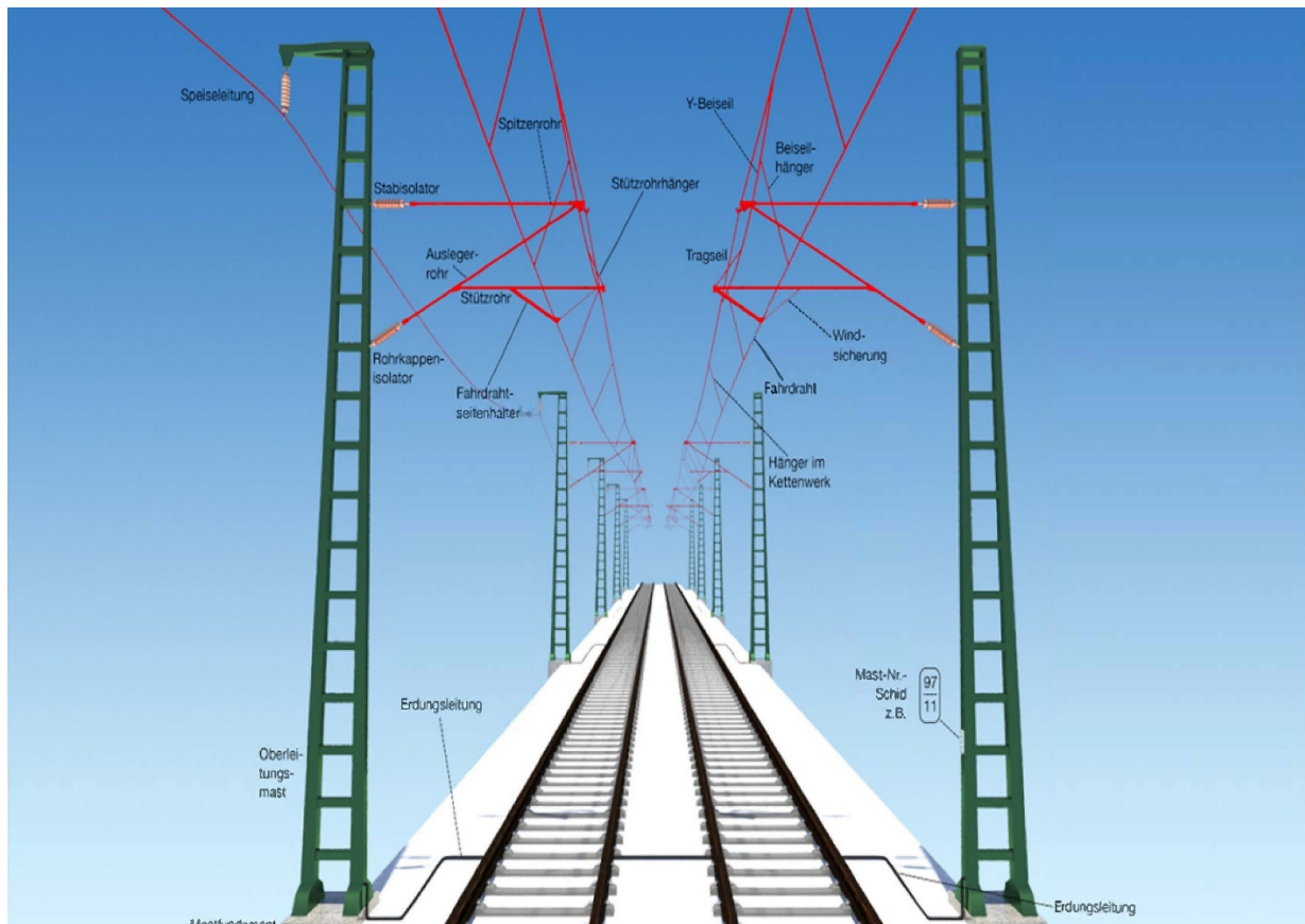
Abbildung 5: Oberleitung mit Einzelaufhängung. Rot kennzeichnet unter Spannung stehende Anlagenteile (Quelle: DB Training)
