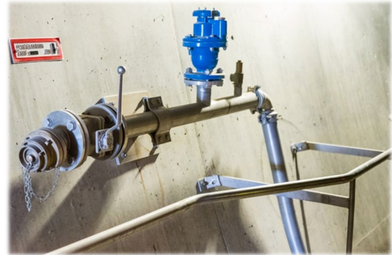
Abbildung 49: Schlauchanschlusseinrichtung
